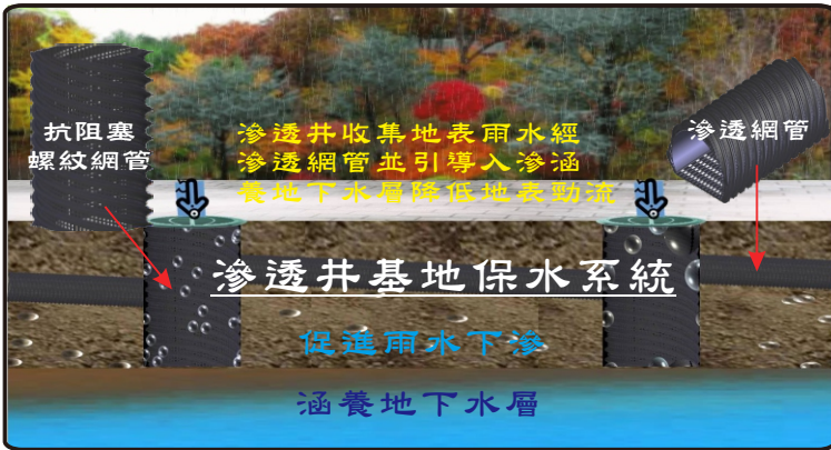
NSO-全透水型
