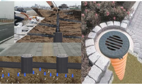
行人步道路面雨水排放
